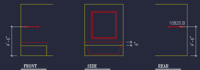
ULTRA BATH TUB DETAILS SCALE: 1/8" = 1'-0"
