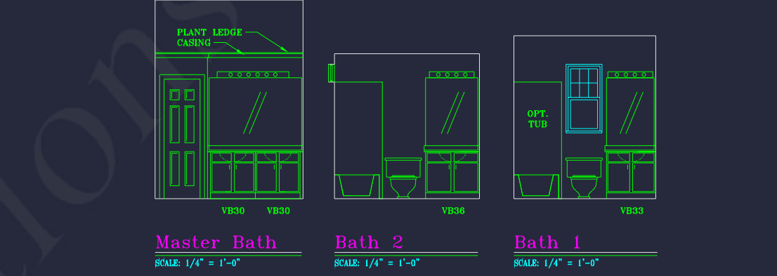
Master Bath SCALE: 1/4" = 1'-0"
