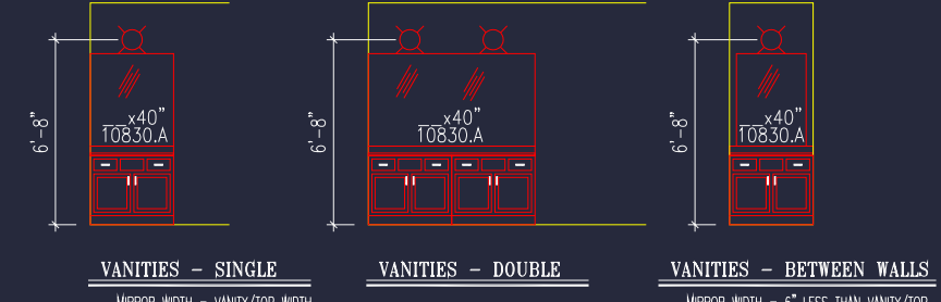
VANITY DETAILS SCALE: 1/8" = 1'-0"
