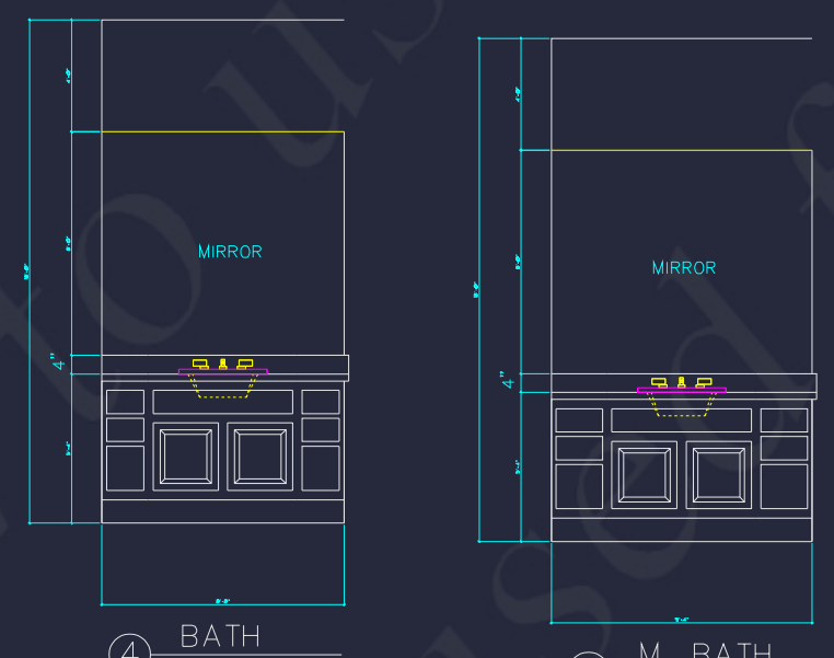
BATH SCALE: 1/4" = 1'-0"
