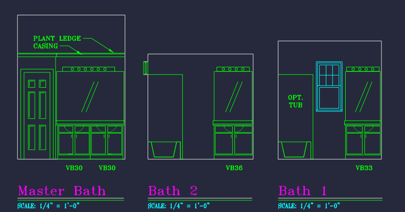
Master Bath SCALE: 1/4" = 1'-0"
