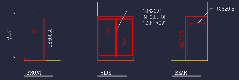
SHOWER DETAILS SCALE: 1/8" = 1'-0"
